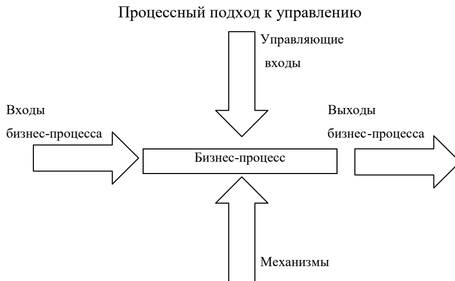
Рисунок 1 - Системный бизнес-процесс
